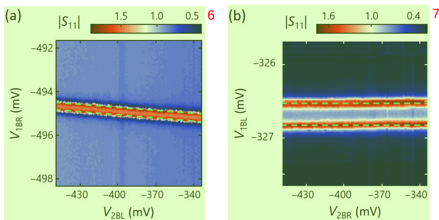
图 5.4 两个双量子点之间的电容串扰。(a) 谐振腔的幅值响应 |S_{11}| 与电极电压 V_{1BR} 和 V_{2BL} 的关系图。(b) 谐振腔的幅值响应 |S_{11}| 与电极电压 V_{1BL} 和 V_{2BR} 的关系图。在图中，我们将探测频率固定在谐振腔频率上。
