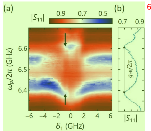
图 5.8 增强真空 Rabi 劈裂。(a) 谐振腔的幅值响应 |S_{11}| 与失谐量 \delta_1 以及探测频率 \omega_p 的关系图。在黑色箭头位置处，发生了增强真空 Rabi 劈裂，产生了两条劈裂宽度为 2g_{\text{eff}}/2\pi = 2 \times 112 \text{ MHz} 的谱线。参数 \delta_1 的扫描方向为从大到小。在 \delta_1 \sim -3 \text{ GHz} 附近，比特 2 的频率发生了抖动，因此图像不再中心对称。(b) 在图 (a) 黑色箭头处截取得到的谐振腔频谱图。
