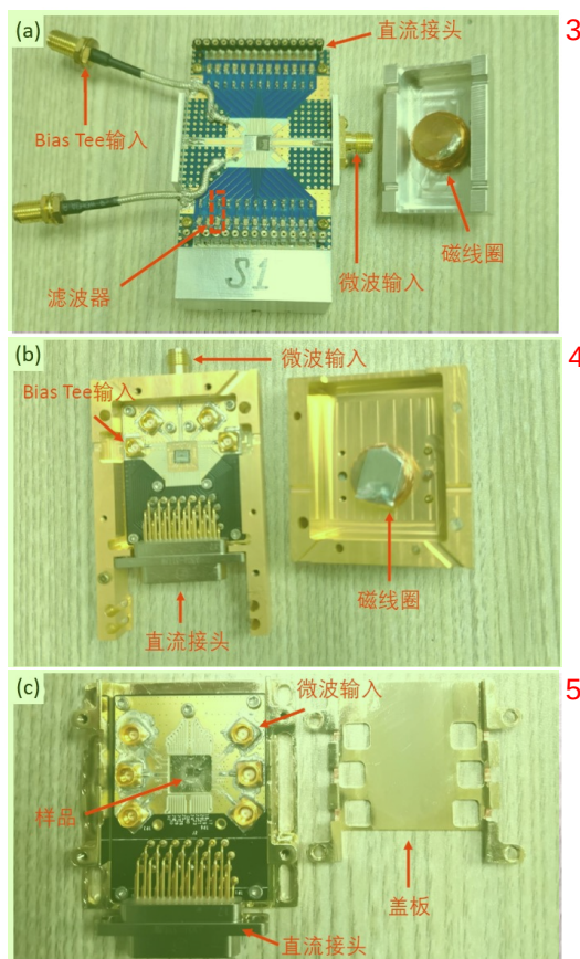
图 2 用于芯片封装的样品盒。(a)-(c) 依次为第一代、第二代以及第三代样品盒。图片引用 6 自 [6].
