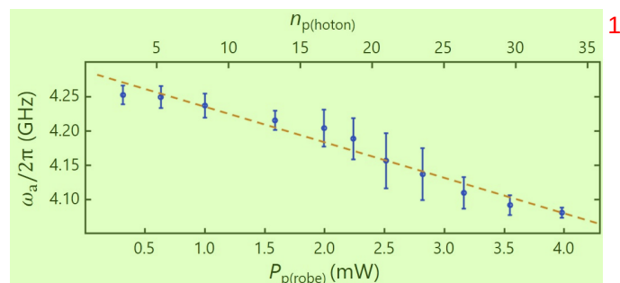
图 3.10 利用比特在色散作用下的频率改变表征谐振腔内光子数与探测微波功率之间的关系。
