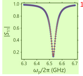
图 3.3 谐振腔反射谱。谐振腔的反射率 |S_{11}| 随着探测频率 \omega_p/2\pi 的变化而变化，并在谐振腔（共振）频率 \omega_r/2\pi = 6.53 GHz 处达到最小值。图中蓝色的圆圈为实验数据，红色的曲线为拟合得到的曲线。该数据已经扣除了本底信号。
