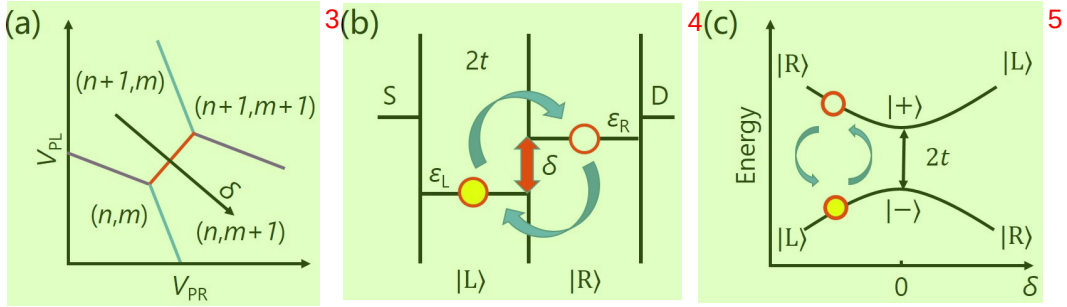
图 2.4 电荷量子比特。(a) 电荷稳态分布示意图。该图是图2.3(c)的局部放大图。在图中红线所示处，量子点间的失谐量为 0，电子持续地在左点与右点之间进行跃迁。(b) 双量子点内电子跃迁示意图。 2t 为双量子点中电子的点间隧穿速率。 \delta 是双量子点之间的失谐量，为左右量子点电势之差 \epsilon_L - \epsilon_R 。(c) 双量子点电荷态能级图。二能级的能量以及成分随着失谐量 \delta 的改变发生变化。
