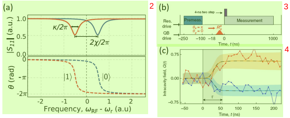
图 4.1 (a) 谐振腔性质与比特状态的色散关系。 \omega_{RF} 为探测微波的频率， \omega_r 为谐振腔的频率。(b) 单发色散读出的波形示意图。(c) 单发读出过程中，测量信号的正交分量 Q 随时间的演化关系图。其中蓝色代表比特处于基态的情况，红色代表比特处于激发态的情况。折线展示了某一次单发读出的演化轨迹，实线展示了将多次单发读出结果平均后得到的轨迹，虚线代表理论计算的结果，而填色区域的宽度展示了在特定时刻正交分量 Q 的标准差。其中，图片 (a) 来自于 [19]，图片 (b) 和 (c) 来自于 [20]。
