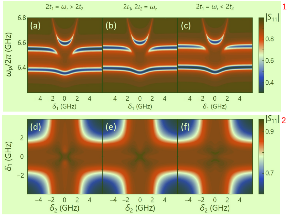
图 5.10 (a)-(c) 增强真空 Rabi 劈裂与 (d)-(f) 两比特关联谱模拟图。其中, (a) 和 (d) 中 2t_2 = 6.46 GHz, (b) 和 (e) 中 2t_2 = 6.48 GHz, (c) 和 (f) 中 2t_2 = 6.50 GHz。在进行模拟计算时, 两比特的耦合强度均为 85 MHz, 退相干速率为 22 MHz。
