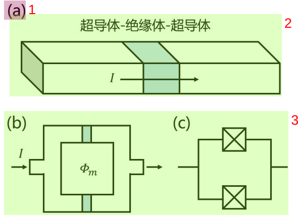
图 2.9 (a) 约瑟夫森结结构示意图。(b) 超导量子干涉仪 (SQUID) 结构示意图。它由两个约瑟夫森结并联形成, \Phi_m 为穿过 SQUID 中间环路部分的磁通大小。(c) 超导量子干涉仪的简化电路示意图。
