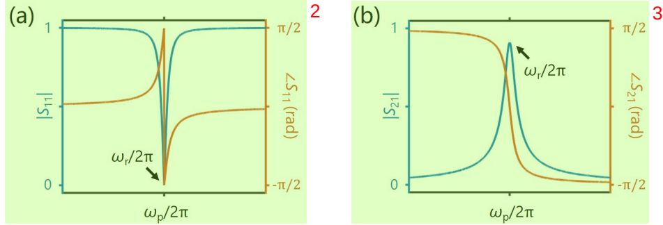
图 2.8 谐振腔的幅值谱与相位谱示意图。(a) 反射式谐振腔。(b) 透射式谐振腔。
