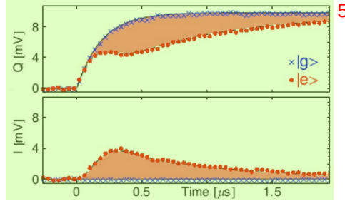
图 4.2 利用主方程模拟得到的测量信号轨迹与实验数据的对比图。图片自于 [21]。 6
