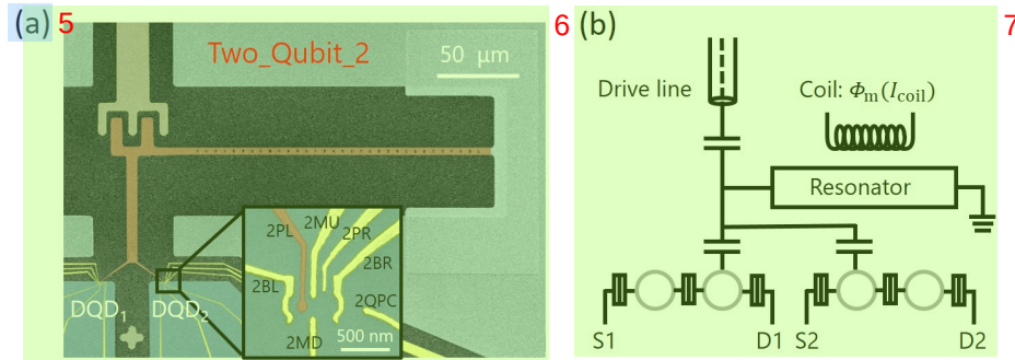
图 5.1 微波谐振腔与半导体量子点集成芯片的结构示意图，编号 Two_Qubit_2。(a) 样品在光镜下拍摄的照片（伪色）。其中，米色部分为传输线，红色部分为高阻抗 SQUID 阵列谐振腔，黄色部分为两个双量子点使用的金属电极，淡蓝色部分为谐振腔的地平面。其中，内插图为右侧量子点的局部放大图，是通过扫描电子显微镜照片拍摄的（伪色）。(b) 样品电路示意图。其中，谐振腔的频率通过悬挂在样品盒上的磁线圈控制。我们通过改变通过磁线圈内部的电流大小 I_{\text{coil}} 来调节通过 SQUID 的磁通大小 \Phi_m 。
