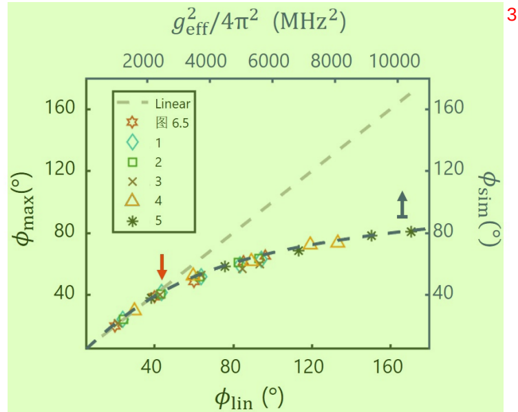
图 6.7 集体微波响应由线性转为非线性的现象。其中， \phi_{\text{lin}} = \sum_k \phi_k 为各个 DQD 最大微波相位响应之和。灰色的虚线为线性估计下的集体微波响应，它满足公式 \phi_{\text{max}} = \phi_{\text{lin}} 。深蓝色的虚线模拟了一个耦合到谐振腔上的激发子在不同耦合强度 g_{\text{eff}} 下对谐振腔相位 \phi_{\text{sim}} 的影响。它的频率为 \omega_{\text{eff}}/2\pi = 5.7 \text{ GHz} ，退相干速率为 \gamma_{\text{eff}}/2\pi = 50 \text{ MHz} 。相位移动 \phi_{\text{sim}} 是根据公式 S_21 = \frac{A_0}{g_{\text{eff}}\chi_{\text{eff}} + \kappa/2} 计算得出的。从图中我们可以看出，线性近似在 \phi_{\text{lin}} \sim 45^{\circ} 或 (g_{\text{eff}}/2\pi)^2 = 55^2 \text{ MHz}^2 (这两个位置满足 \sum_k g_k \chi_k = g_{\text{eff}}\chi_{\text{eff}} \sim \kappa/2 ) 开始与实验现象明显不符。
