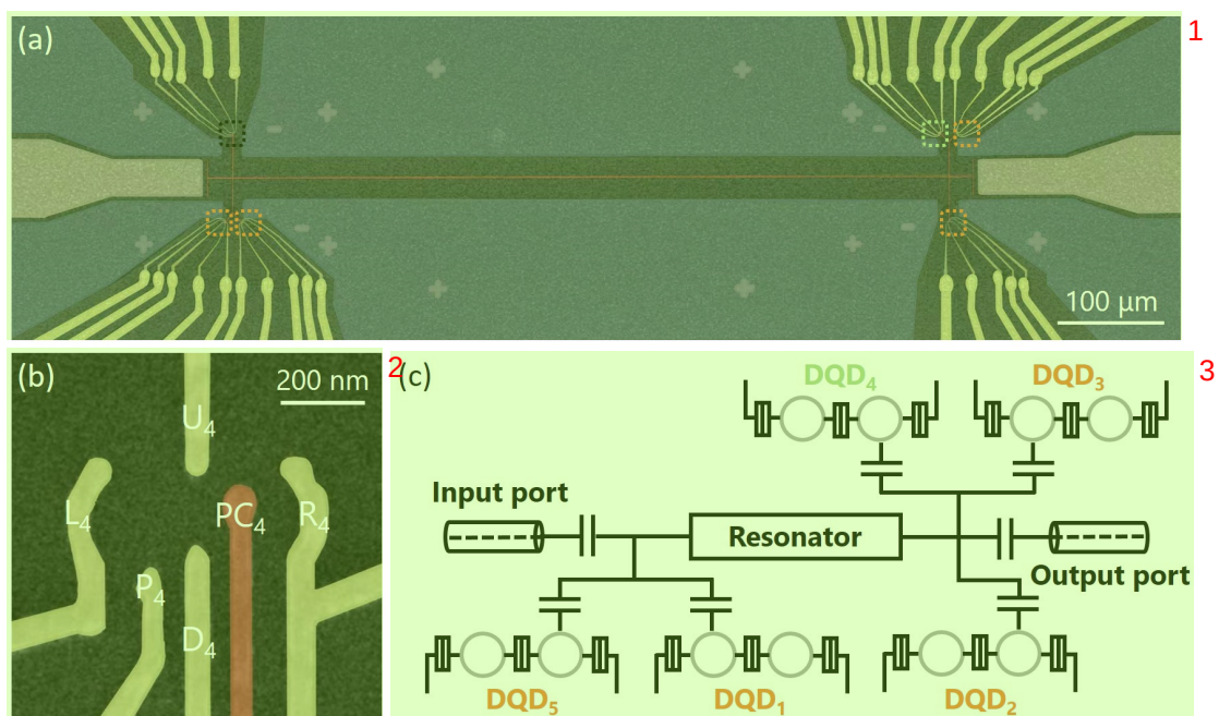
图 6.1 样品的扫描电子显微镜照片（伪色）(a) 超导微波谐振腔（红色）通过电容与外界传输线（米色）耦合，并且在每个电压波腹位置耦合了三个双量子点。图中的虚线方框标记了六个双量子点的位置，其中黑色方框标记那个双量子点无法正常工作。(b) DQD_4 电极结构放大图。它的位置在图 (a) 中由绿色虚线方框展示。(c) 样品的简化电路图。在实验中，我们的探测微波将由输入端口（input port）进入谐振腔，然后测量从输出端口（output port）透射而出的微波信号。
