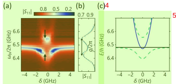
图 3.7 真空 Rabi 劈裂。数据来自与样品 Two_Qubit_2 中左侧的双量子点。(a) 受电荷比特调制的谐振腔频谱图。在黑色箭头位置处，比特频率与谐振腔频率相等并发生真空 Rabi 劈裂，产生了两条劈裂宽度为 2g/2\pi = 2 \times 81 MHz 的谱线。(b) 在图 (a) 黑色箭头处截取得到的谐振腔频谱图。图中的红色实线为式3.1的拟合曲线。我们注意到，在比特与光子共振时，它们形成了最大杂化态，两条谱线对应的线宽一致，为比特线宽和谐振腔线宽的算术平均值 [1,20-21] 。(c) 利用 J-C 模型模拟的杂化系统能级图。其中黑色实线与蓝色实线分别为未发生耦合时光子与比特的能级，而绿色虚线为发生耦合后杂化系统的能级。模式所用到的参数为隧穿速率 2t/2\pi = 6.47 GHz、谐振腔频率 \omega_r = 6.48 GHz、电荷比特与光子的耦合强度为 g/2\pi = 81 MHz。
