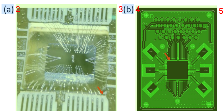
图3 (a) 完成与电路板线路连接的芯片。(b) 第三代样品盒所使用电路板的示意图。
