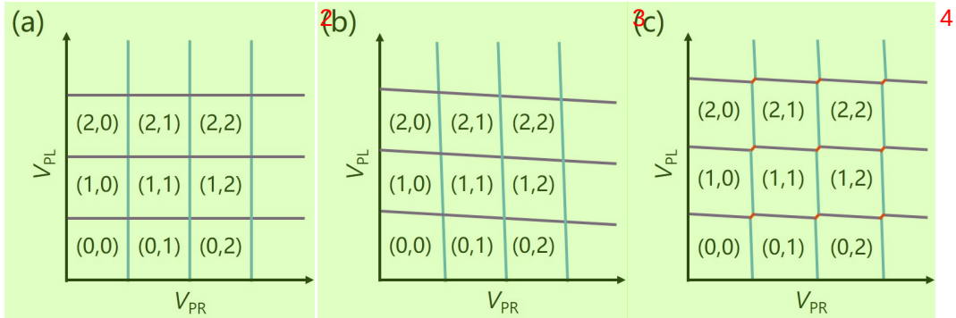
图 2.3 电荷稳态分布图。(a) 量子点器件无寄生电容，且量子点之间的耦合电容 C_M 为 0 的情况。(b) 量子点器件存在寄生电容，而量子点之间的耦合电容 C_M 为 0 的情况。(c) 量子点器件存在寄生电容，且量子点之间的耦合电容 C_M 不为 0 的情况。其中， (n, m) 分别代表了左点和右点内的电子数目。
