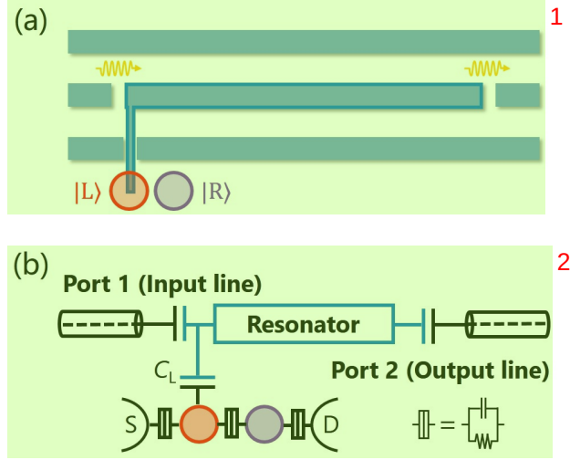
图 2.15 集成了单个双量子点的共面波导谐振腔。(a) 样品结构示意图。(b) 样品电路示意图。
