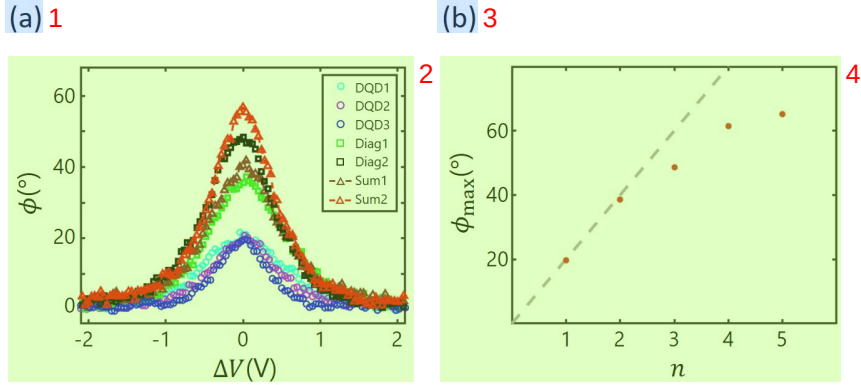
图 6.6 受多个比特调制的集体微波响应。(a) 实际测量得到的集体微波响应与线性估计的集体微波响应之间的对比图。其中，来自 \text{DQD}_{1(2)} 的单比特的微波响应（图中的亮蓝色（紫色）圆圈）是沿图6.5(a)中的 y ( x ) 轴截取而来的，而来自 \text{DQD}_3 的单比特的微波响应（图中的深蓝色圆圈）则是沿图6.5(b)中的 x 轴截取而来的。绿色（黑色）方块为两（三）比特情况时的集体微波响应，它们是沿着图6.5(a)[图6.5(b)] 中红色虚线截取出来的数据。棕色（红色）三角为前两（三）个比特的独立微波响应之和。(b) 从图6.5中提取的最大相位位移量 \phi_{\max} 与参与耦合的比特数目 n 之间的依赖关系。其中，灰色的虚线为线性估计下的集体微波响应，它满足公式 \phi_{\max} = 20n 。
