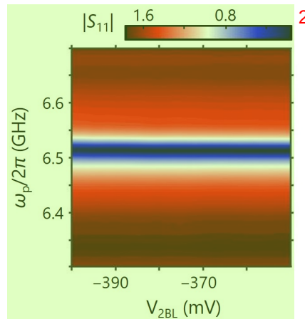
图 5.5 电极电压对谐振腔谐振频率的干扰。谐振腔的幅值响应 |S_{11}| 与电极电压 V_{2BL} 以及探测频率 \omega_p 的关系图。此时，两个量子点均未成型，谐振腔的频率略大于我们在实验中使用的 \omega_r/2\pi = 6.48 \text{ GHz} 。
