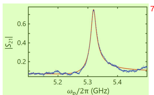
图 6.2 谐振腔透射谱。其中，蓝色的原点为实验数据，红色的实线为拟合曲线。 8
