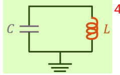
图 2.5 LC 谐振器电路图。
