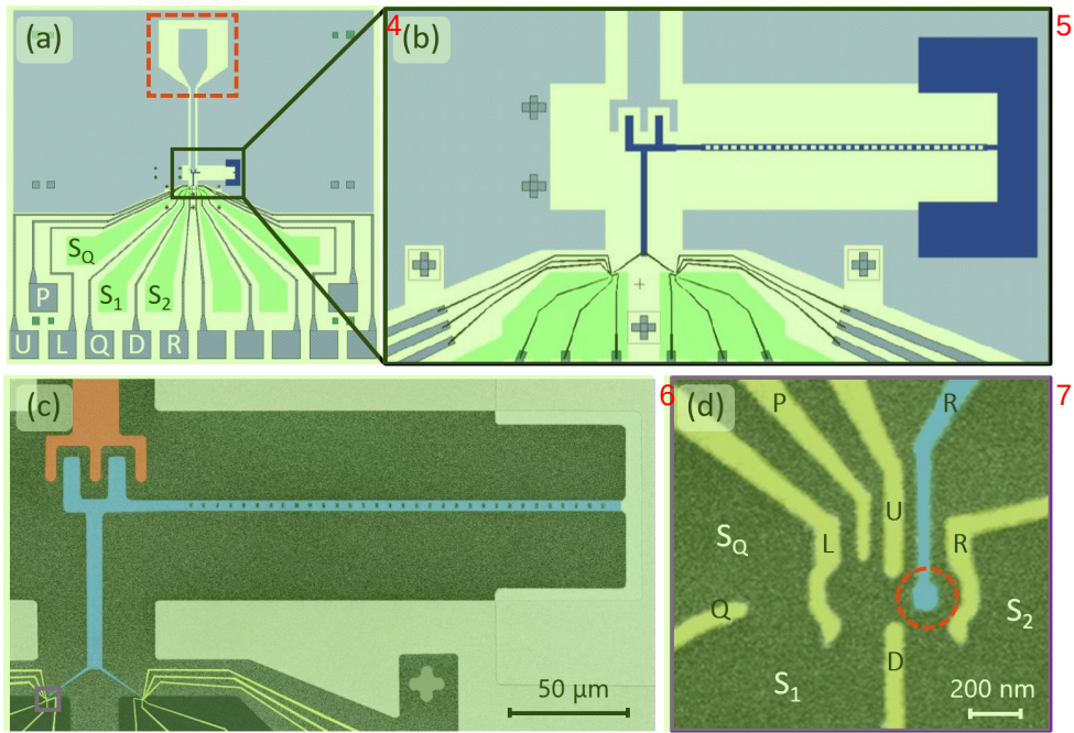
图 1 微波谐振腔与半导体量子点集成芯片的结构示意图。 4 (a) 高阻抗 SQUID 阵列谐振腔与两个双量子点耦合样品的结构设计图。该芯片的整体尺寸为 3 \times 3 \text{ mm}^2 。在该图中，我们标记了左侧量子点使用的电极。其中，电极 P、U、L、D、R 用于控制双量子点性质（节 2.1.2）；电极 Q 被用于量子点接触（quantum point contact, QPC）；电极 S_1 与 S_2 为量子点的源漏电极；电极 S_Q 配合 S_1 可以用于测量量子点接触的电流。 5 (b) 为图 (a) 中谐振腔区域的放大图。深蓝色部分从左到右可以分为三个结构，即用于耦合两个量子点以及外部传输线的电极结构、提供高电感的 SQUID 阵列、用于形成地平面的大电容结构。 6 (c) 高阻抗 SQUID 阵列谐振腔与两个双量子点耦合样品的扫描电子显微镜照片（伪色）。其中，红色部分为传输线，蓝色部分为 SQUID 阵列谐振腔，黄色部分为两个双量子点使用的金属电极，银色部分为谐振腔的地平面。由紫色方框圈中的部分为左侧的双量子点。 7 (d) 左侧双量子点的扫描电子显微镜照片（伪色）。
