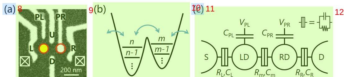
图 2.2 门控双量子点。(a) 门控双量子点的扫描电子显微镜照片。红圈表示两个量子点的形成位置。(b) 双量子点的束缚势示意图。在两侧势阱中都存在数个分立的能级，电子可越过中间的势垒在两个量子点之间跃迁。同时，电子也可以在源漏电子库以及量子点之间跃迁。(c) 双量子点的等效电路图。电子处于左量子点 (LD) 以及右量子点 (RD) 之中。两侧源漏电子库分标记为 S 和 D。其中，隧穿势垒由电阻与电容并联构成，其电容大小受对应电极上的偏置电压控制。
