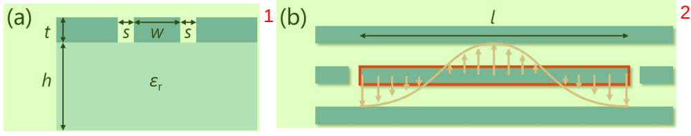
图 2.6 共面波导谐振腔示意图。(a) 共面波导传输线的横截面示意图。其中，中心导体宽度为 w ，中心导体与两侧地平面的间隔为 s ，膜的厚度为 t 。而在共面波导传输线结构下方的基片厚度为 h ，相对介电常数为 \varepsilon_r 。(b) 共面波导透射腔结构的示意图。中间由红色方框所示的为透射腔部分，与两端的传输线存在电容耦合。电磁场在谐振腔内形成驻波，图中使用粉红色标图图形为谐振腔内产生的全波长驻波示意图。
