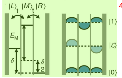
图 2.17 串联三量子点能级示意图。左图展示了该系统的能级结构。右侧展示了系统中三个本征态对应在各个点中的分部概率。图片引用自 [76] 。
