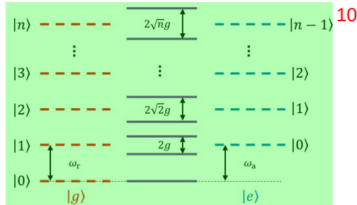
图 2.13 二能级原子与谐振腔共振 ( \Delta = 0 ) 时, Jaynes-Cummings 哈密顿量的能级示意图。 11 红色 (蓝色) 虚线代表两子系统不存在耦合时, 原子处于基态 |g\rangle ( |e\rangle ) 且光子数态为 |k\rangle 时的系统能级。紫色实线代表在相互作用下形成的新本征能级。
