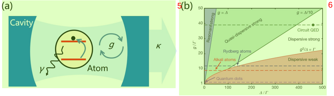
图 2.12 (a) 二能级原子与谐振腔内光场的相互作用示意图。二能级原子的退相干速率为 \gamma ，光子的耗散速率为 \kappa ，两者之间的耦合强度为 g 。(b) 腔量子电动力学参数空间示意图。其中， \Delta 为二能级原子与谐振腔频率之差， \Gamma 为比特退相干速率与光子耗散速率之中的最大值。根据耦合强度与失谐量的大小可将相互作用划分为几个不同的区间。图片引用自 [54]。
