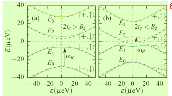
图 2.16 在双量子点中自旋的哈密顿量能级示意图。其中虚线代表 B_x = 0 的情况，即自旋-轨道耦合作用强度为零对应的系统能级。(a) 2t_{(c)} > B_z 的情况。(b) 2t_{(c)} < B_z 的情况该图片引用自 [73]。
