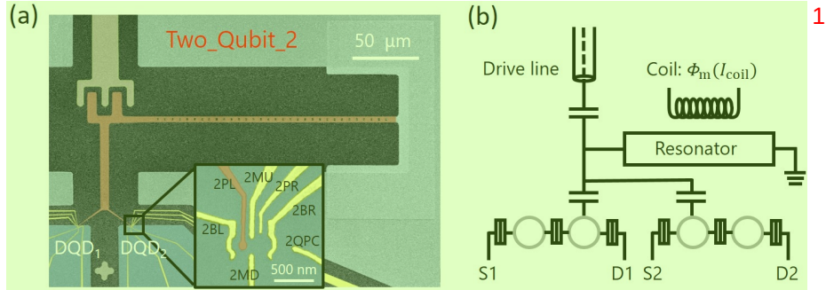
图 3.2 微波谐振腔与半导体量子点集成芯片的。该样品为 Two_Qubit_2。(a) 样品在光镜下拍摄的照片（伪色）。其中，米色部分为传输线，红色部分为 SQUID 阵列谐振腔，黄色部分为两个双量子点使用的金属电极，淡蓝色部分为谐振腔的地平面。其中，内插图图为右侧量子点的局部放大图，是通过扫描电子显微镜照片拍摄的（伪色）。(b) 样品电路示意图。其中，谐振腔的频率通过悬挂在样品盒上的磁线圈控制。我们通过改变通过磁线圈内部的电流大小 I_{coil} 来调节通过 SQUID 的磁通大小 \Phi_m 。
